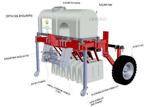
Şekil 2. Yastık ilaçlama ekipmanı - Tasarım modeli teknik çizimi (perspektif görünüm).
